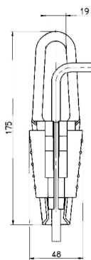
Держатель кабеля
