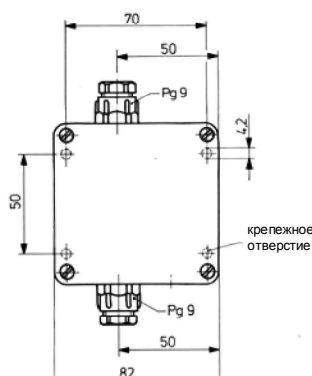
Клеммная коробка с компенсацией давления
