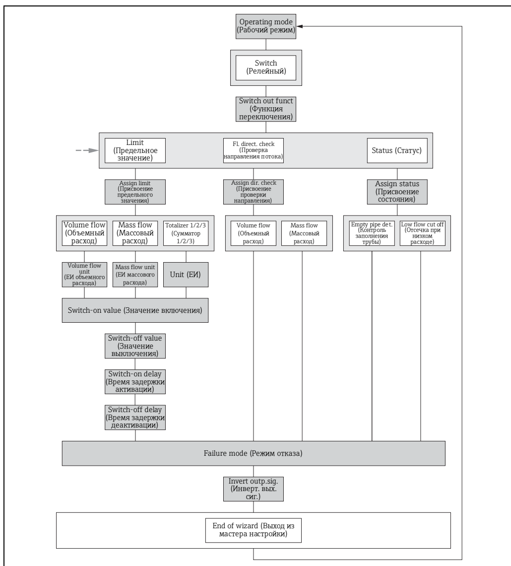
22 Мастер «Pulse/frequency/switch output» (Импульсный/частотный/релейный выход) в меню «Setup» (Настройка): параметр «Operating mode» (Рабочий режим), опция «Switch» (Релейный) (часть 2)
