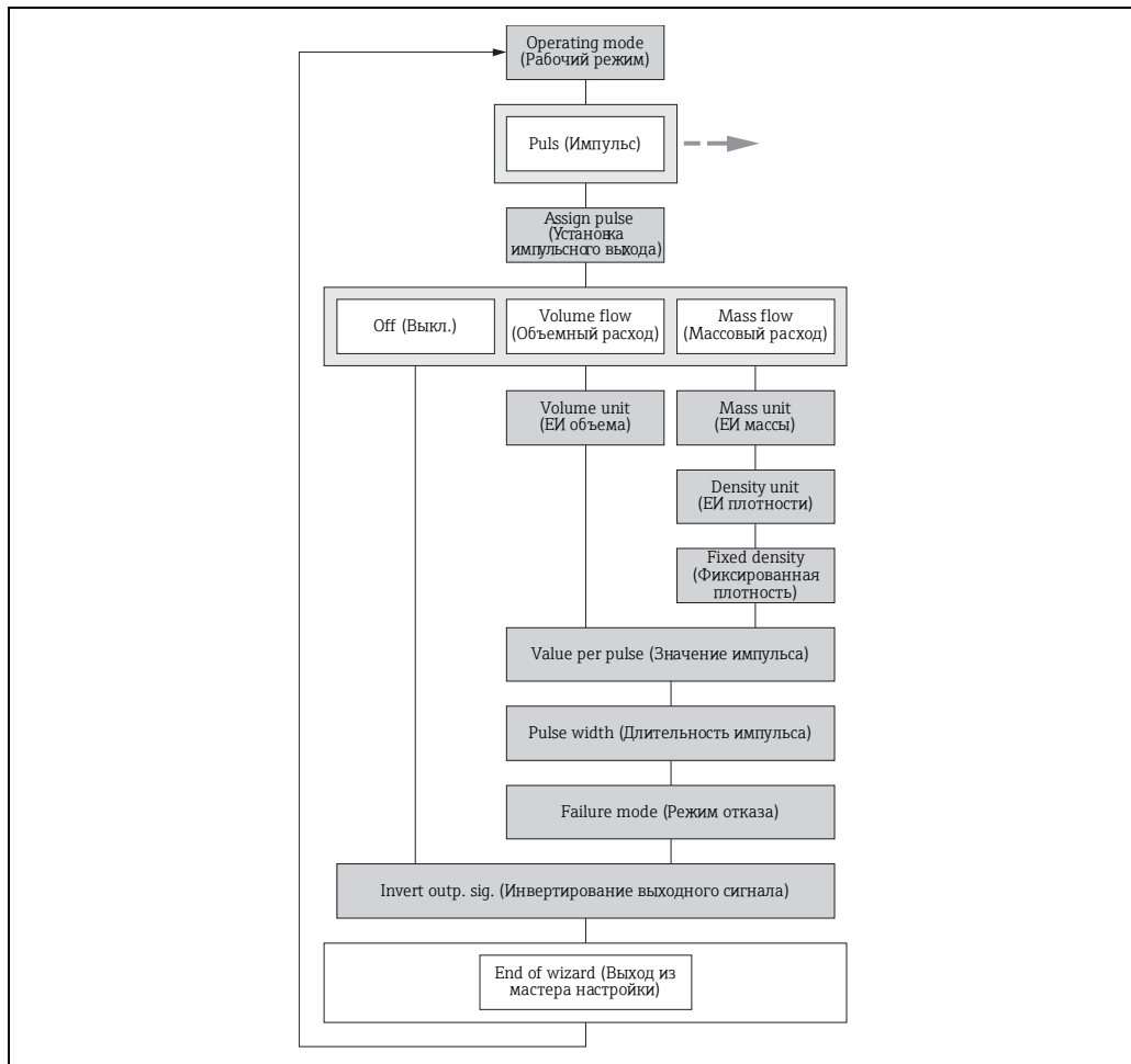
19 Мастер «Pulse/frequency/switch output» (Импульсный/частотный/релейный выход) в меню «Setup» (Настройка): параметр «Operating mode» (Режим работы), опция «Puls» (Импульсный)
