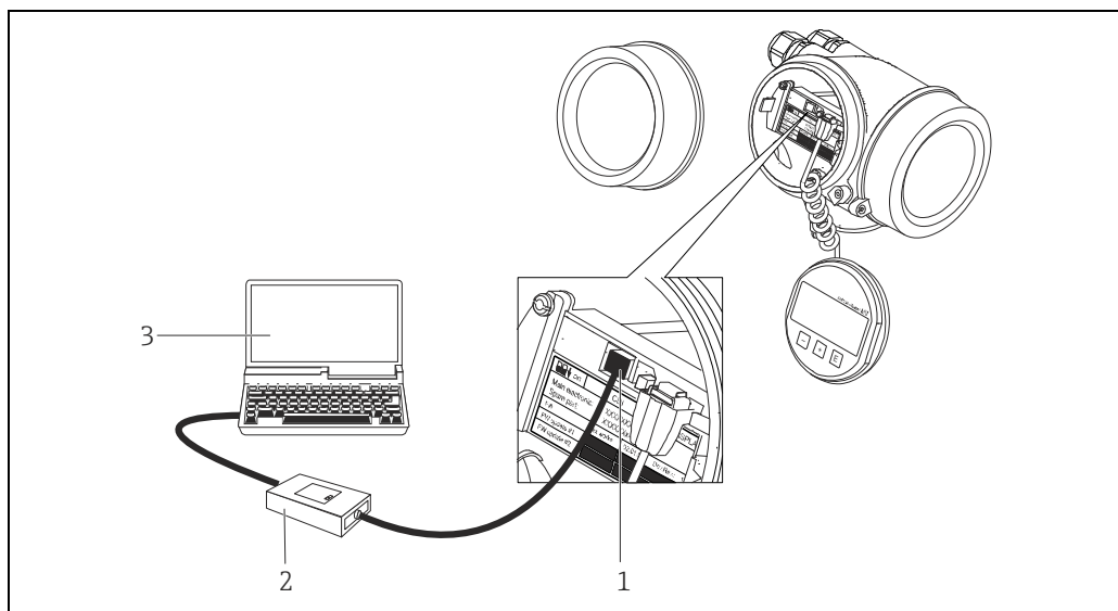
1 Служебный интерфейс (CDI = Common Data Interface, единый интерфейс данных Endress+Hauser) измерительного прибора 2 Коммутирующая коробка FXA291 3 Компьютер с управляющей программой «FieldCare» и COM DTM «CDI Communication FXA291»
