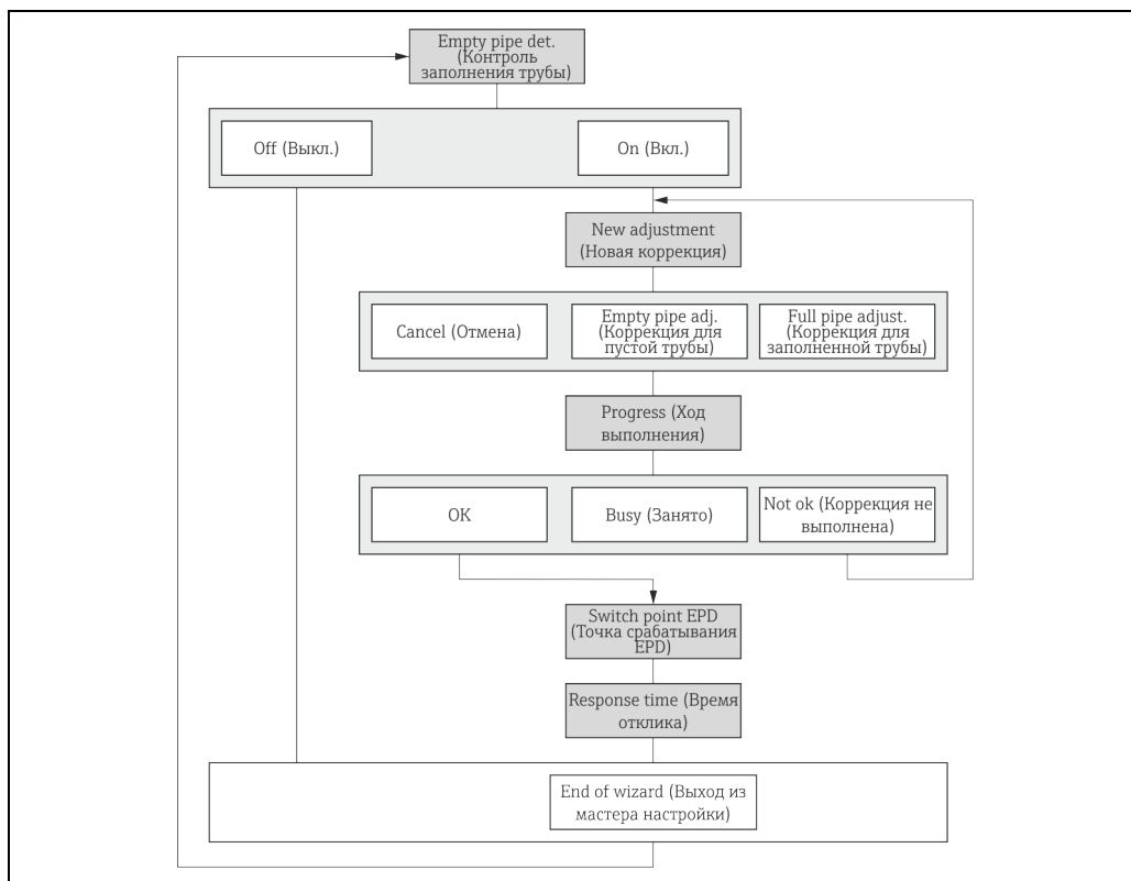
26 Мастер «Empty pipe detection» (Контроль заполнения трубы) в меню «Setup» (Настройка)
