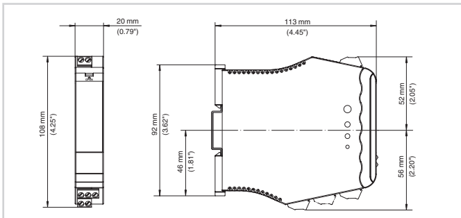
Размеры VEGATOR 111
